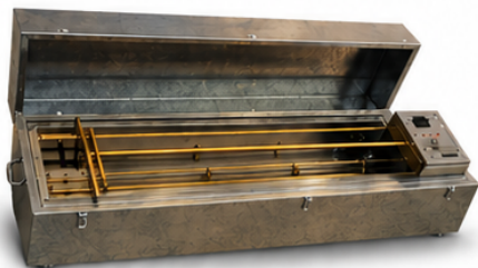
DUCTILÔMETRO E RECUPERADOR ELÁSTICO
