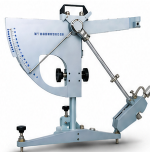
PÊNDULO BRITÂNICO
